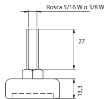
Regatón Ø 36 Cód: 107363/8 -107365/16
