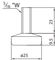
Regatón Ø 25 plano Cód: 10725P
