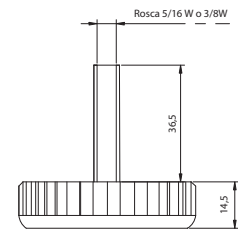
Regatón Ø 55 Cód: 107555/16 -107553/8
