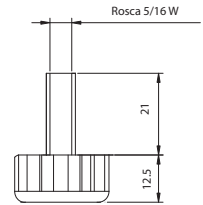
Regatón Ø 25 base alta Cód: 10725BA
